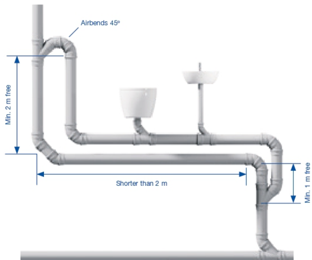
Fig. 24: Bypass pipe conforming to DIN 1986-100.
